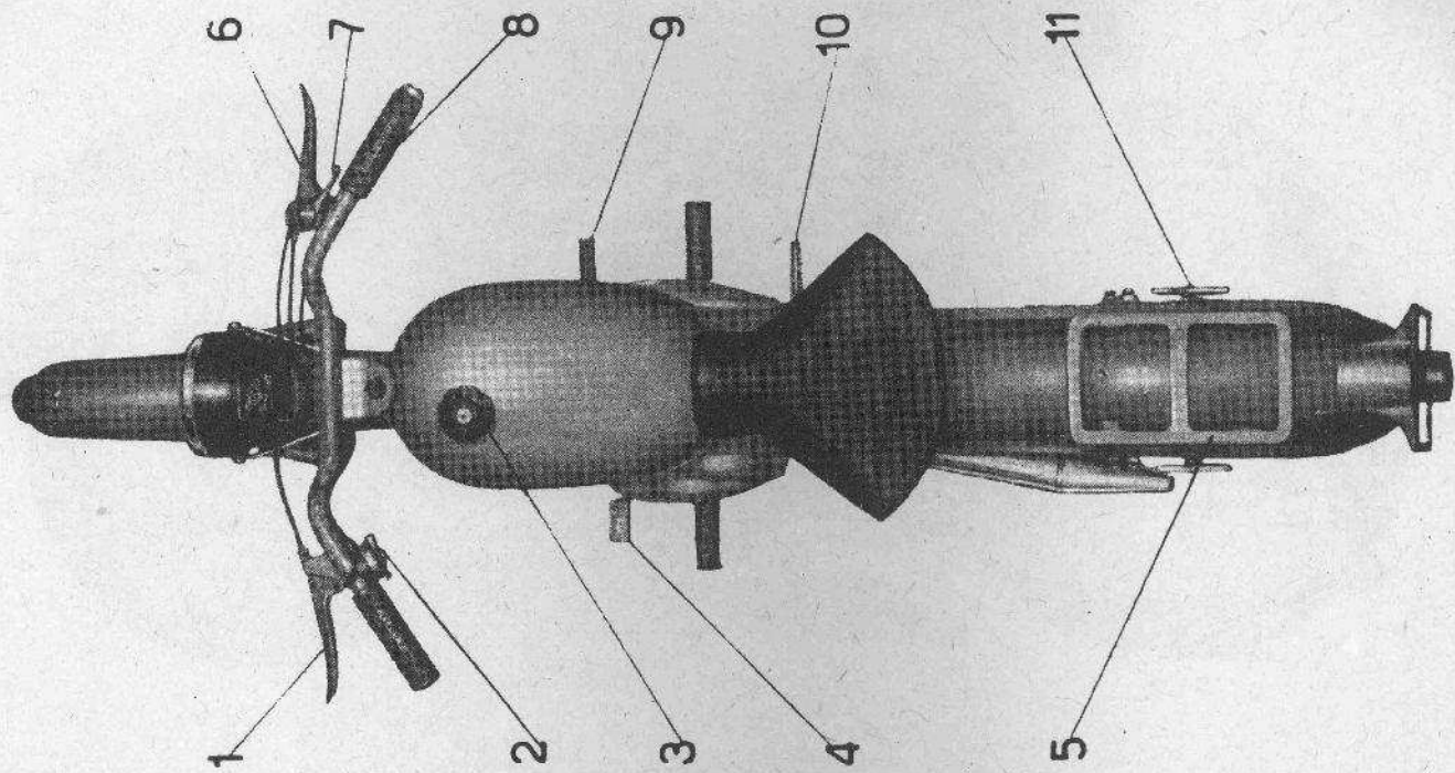
Fig. 3 - (comandi ed accessori)
